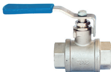
PN40. PASO TOTAL. PRENSA ESTOPA EN EL EJE. PALANCAS ACERO INOX. SISTEMA ANTIHIELO
