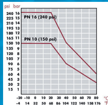
GRAFICO RELACION PRESION-TEMPERATURA
